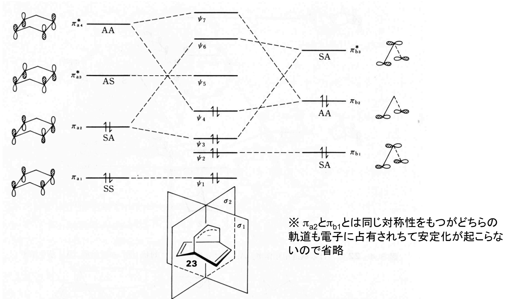
図 3.5 23 における軌道相互作用. \sigma_1 , \sigma_2 に関して対称 (S) か反対称 (A) かをこの順に記してある
